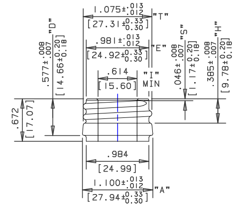
DETALLE DE ACABADO 28-1620-R05 ESC. 1:1
