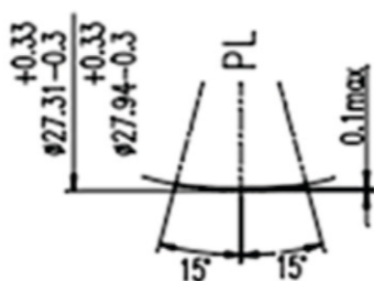
Detalle reducido de boca y tapa de botella 2:1
