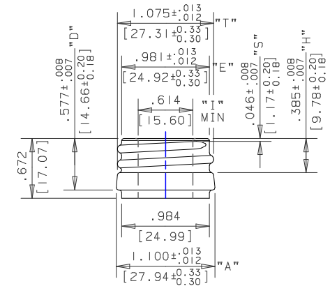
28-1620-R05 ESC. 1:1
